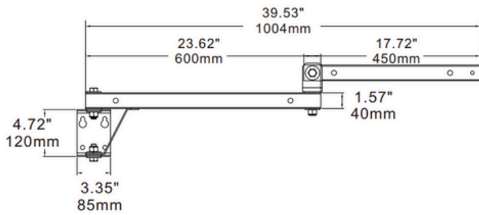
40" Bracket A1
