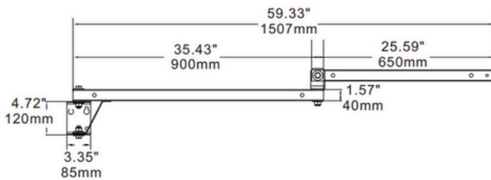
60" Bracket A3
