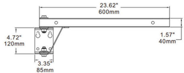
24" Bracket A4
